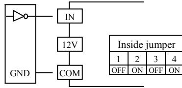
TTL input (5V)
